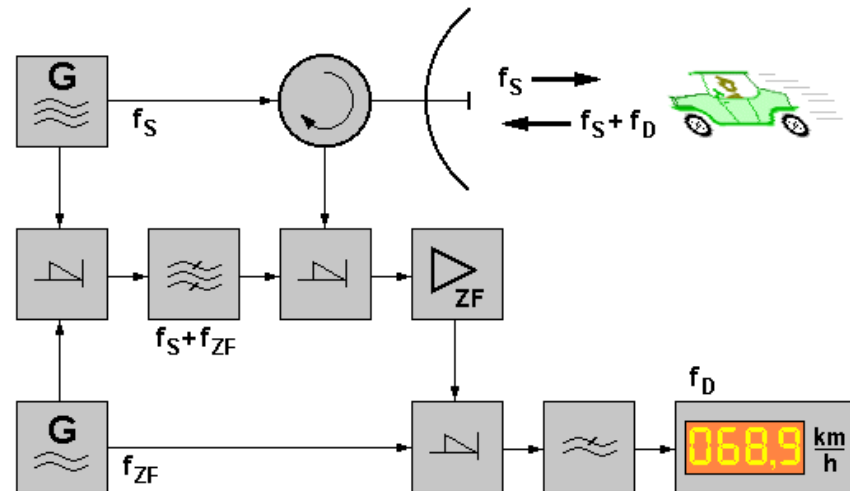
Abb. 5: Blockschaltbild eines einfachen CW-Radars
