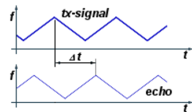
Abb 6: Entfernungsbestimmung durch Laufzeitmessung mit einem FMCW-Radar
